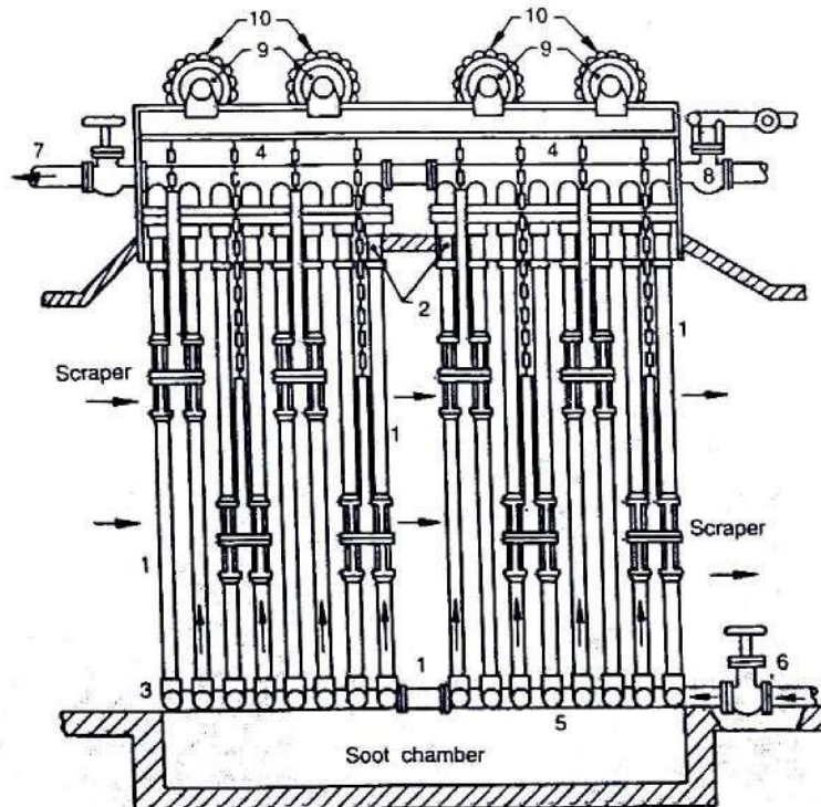
Fig. 3.16 Economiser
